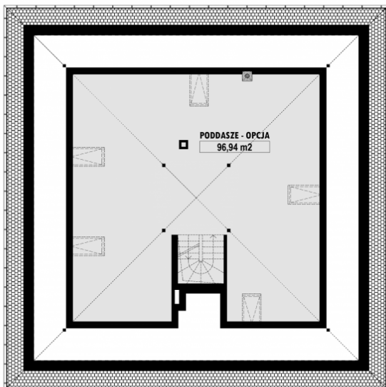
E-230a PODDASZE
