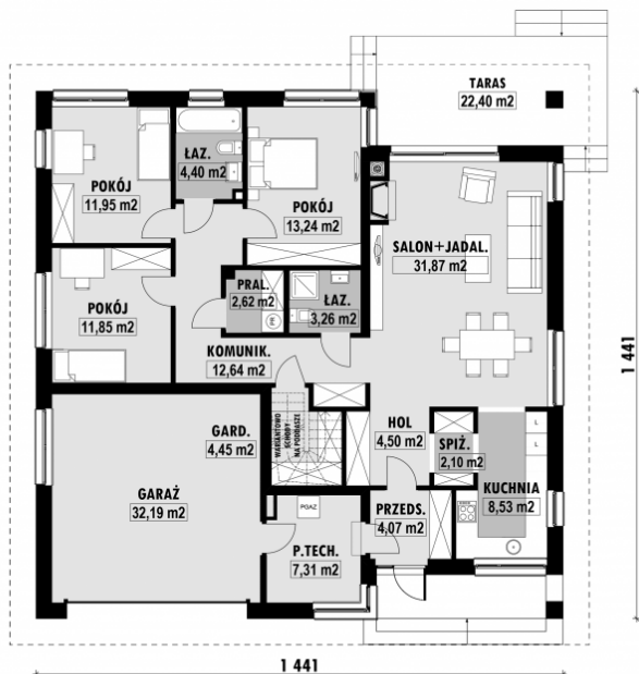
E-230a PARTER
