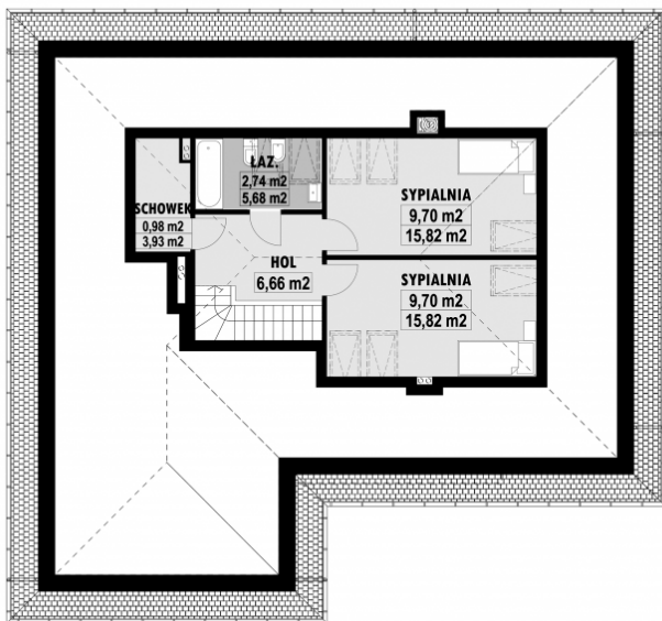
E-134 PODDASZE
