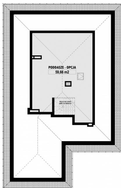
E-121 PODDASZE
